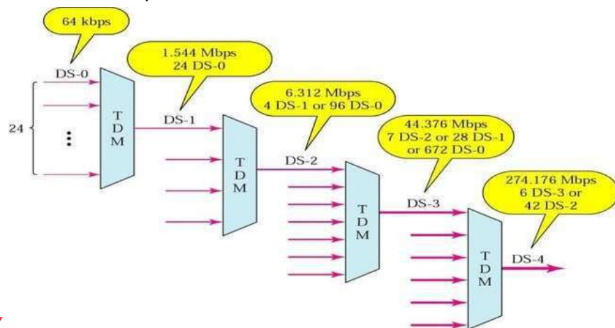
DS-hierarchy
