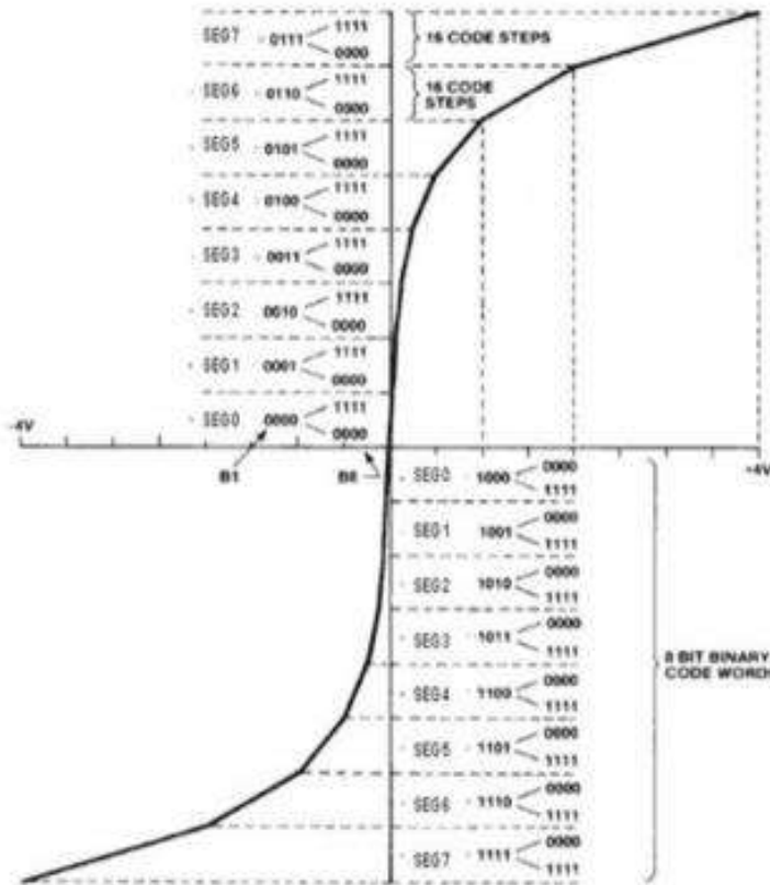
13SegmentScale
